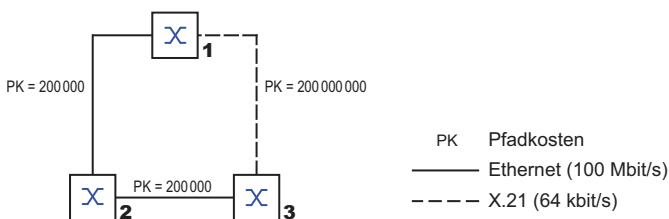
Abb. 34: Pfadkosten
