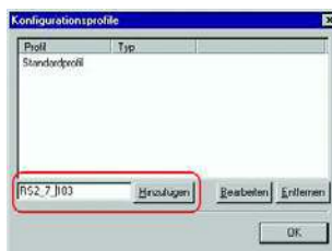
Abb. 59: Konfigurationsprofile hinzufügen
