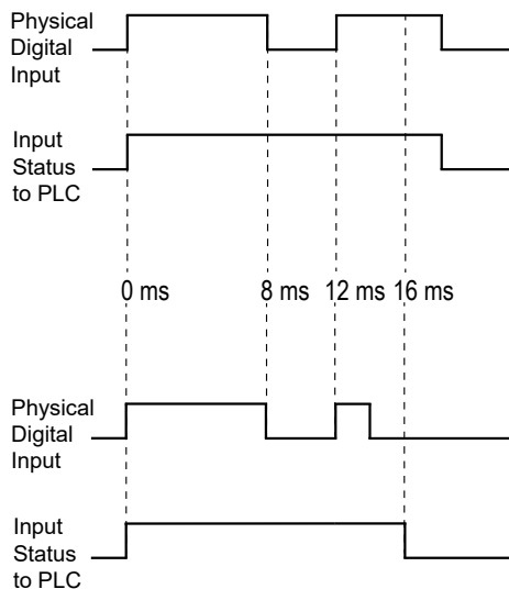
Figure 28: DI Extension
