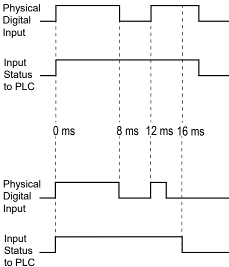
Figure 13: DI Extension
