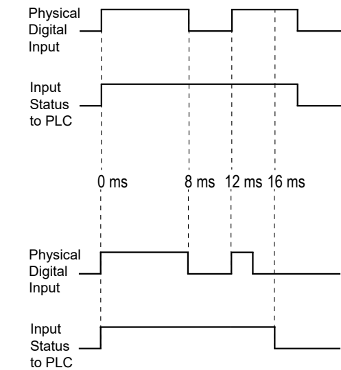
Abb. 13: DI Extension
