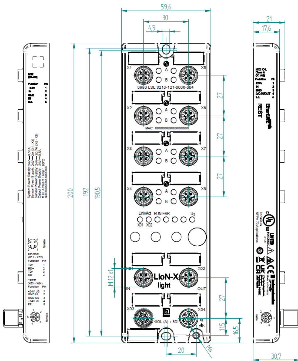
Abb. 7: 0980 LSL 3210-121-0006-004
