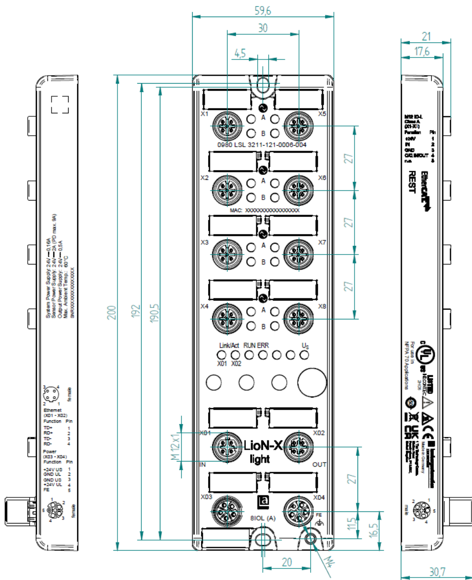
Abb. 6: 0980 LSL 3211-121-0006-004
