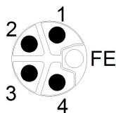
Abb. 9: Schemazeichnung M12 L-Kodierung (Stecker X03 für Power In)
