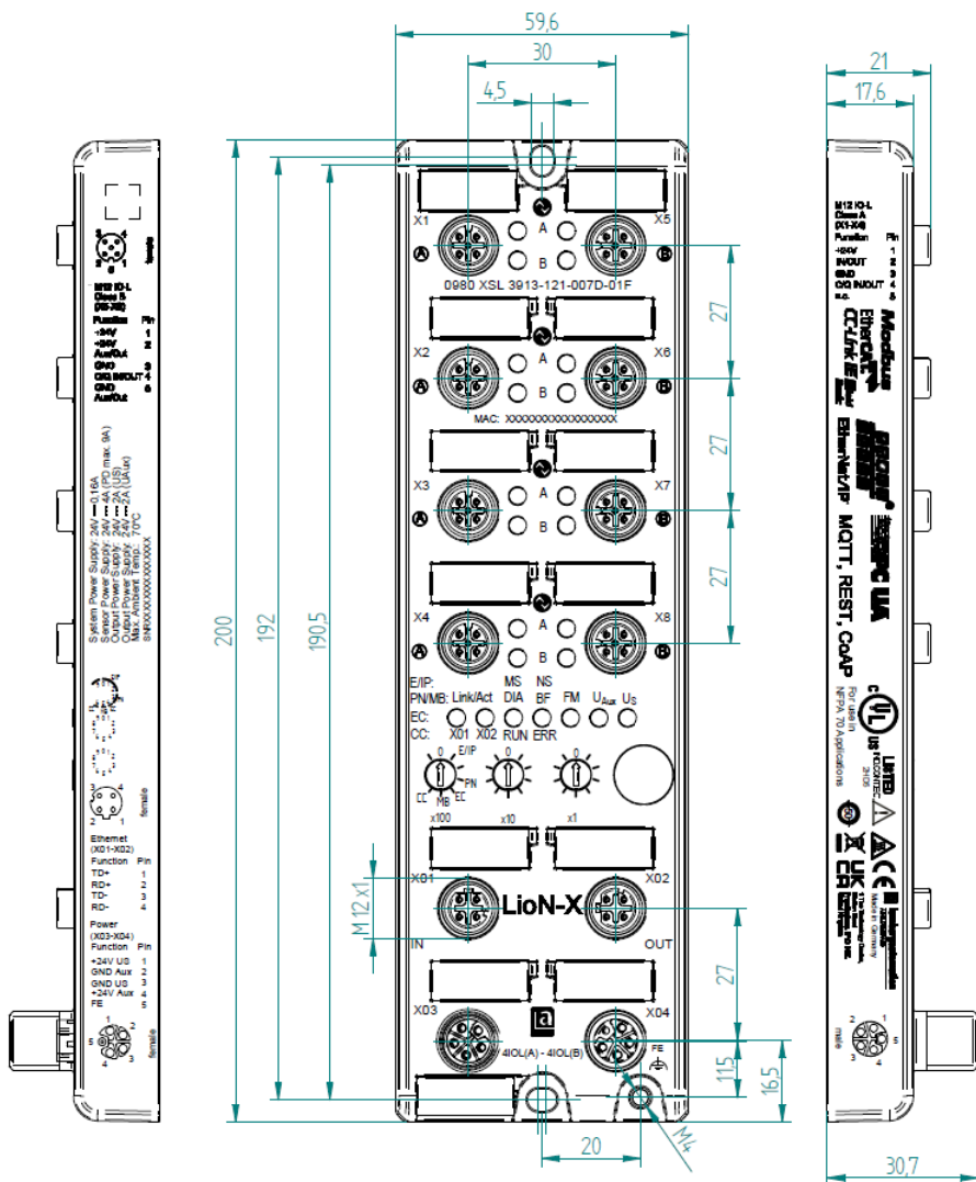
Abb. 4: 0980 XSL 3913-121-007D-01F
