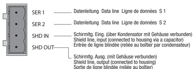
Anschlussbelegung 4poliger Steckverbinder Pin assignment of 4-pin connector Affectation des broches dans le connecteur multibroches à 4 pôles
