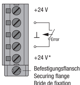
Anschlussbelegung 5poliger Klemmblock Pin assignment of the 5-pole screw clamp block Mode de raccordement sur le bloc à vis à 5 pôles
