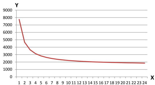
Figure 27 SAToP, CESoPSN Bandwidth
