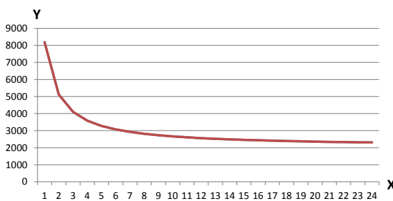
Figure 27 SAToP, CESoPSN Bandwidth
