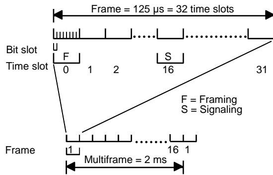
Figure 6 E1 Framing
